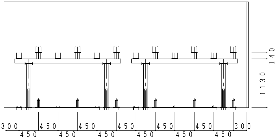
立面図
