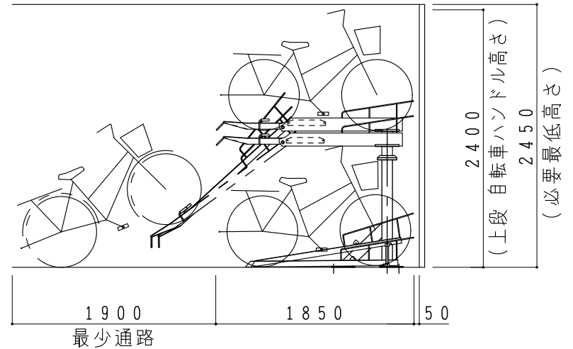
側面図
