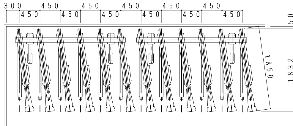
平面図
