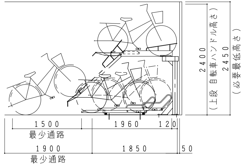
側面図
