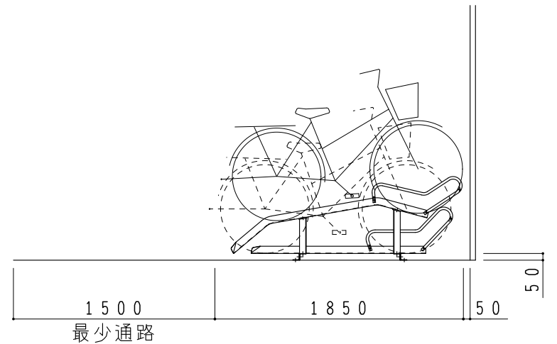
側面図
