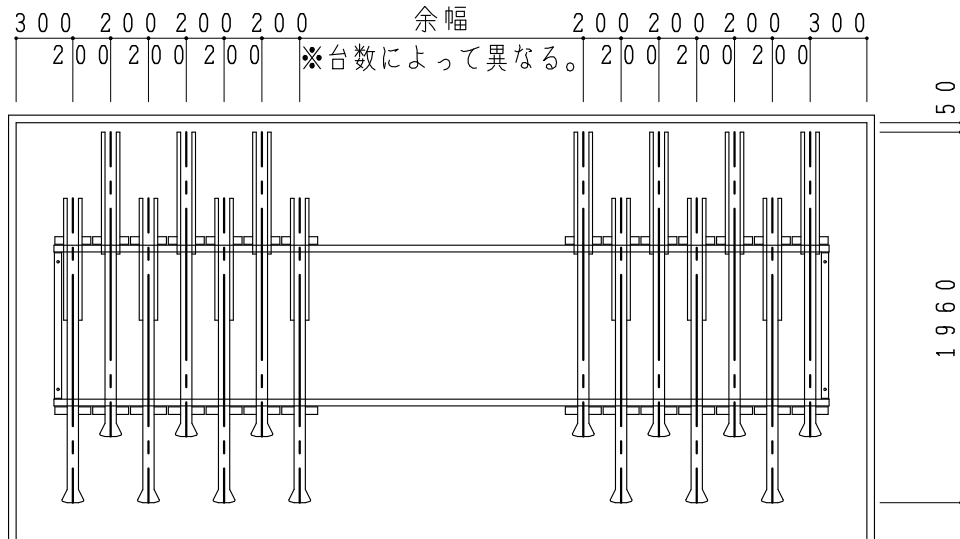
平面図
