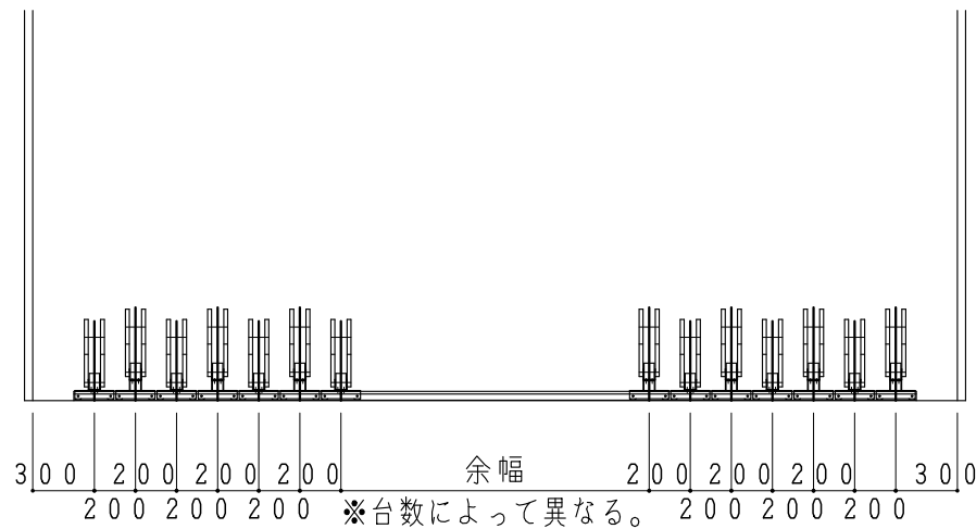
立面図
