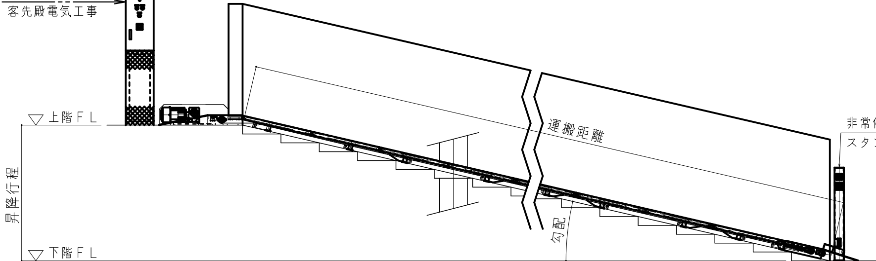
側面図
