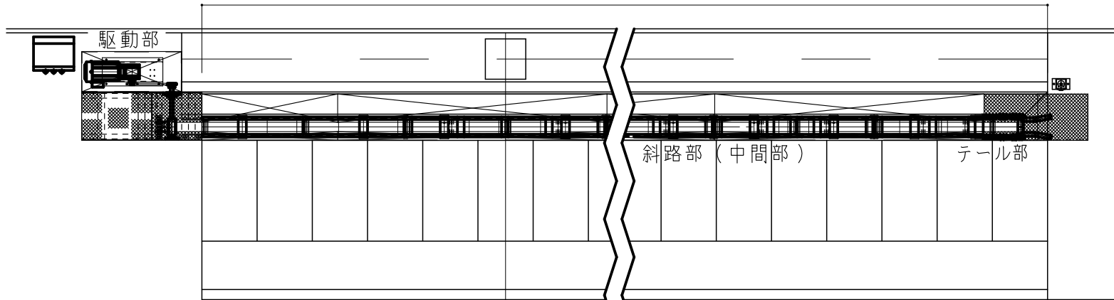
平面図
